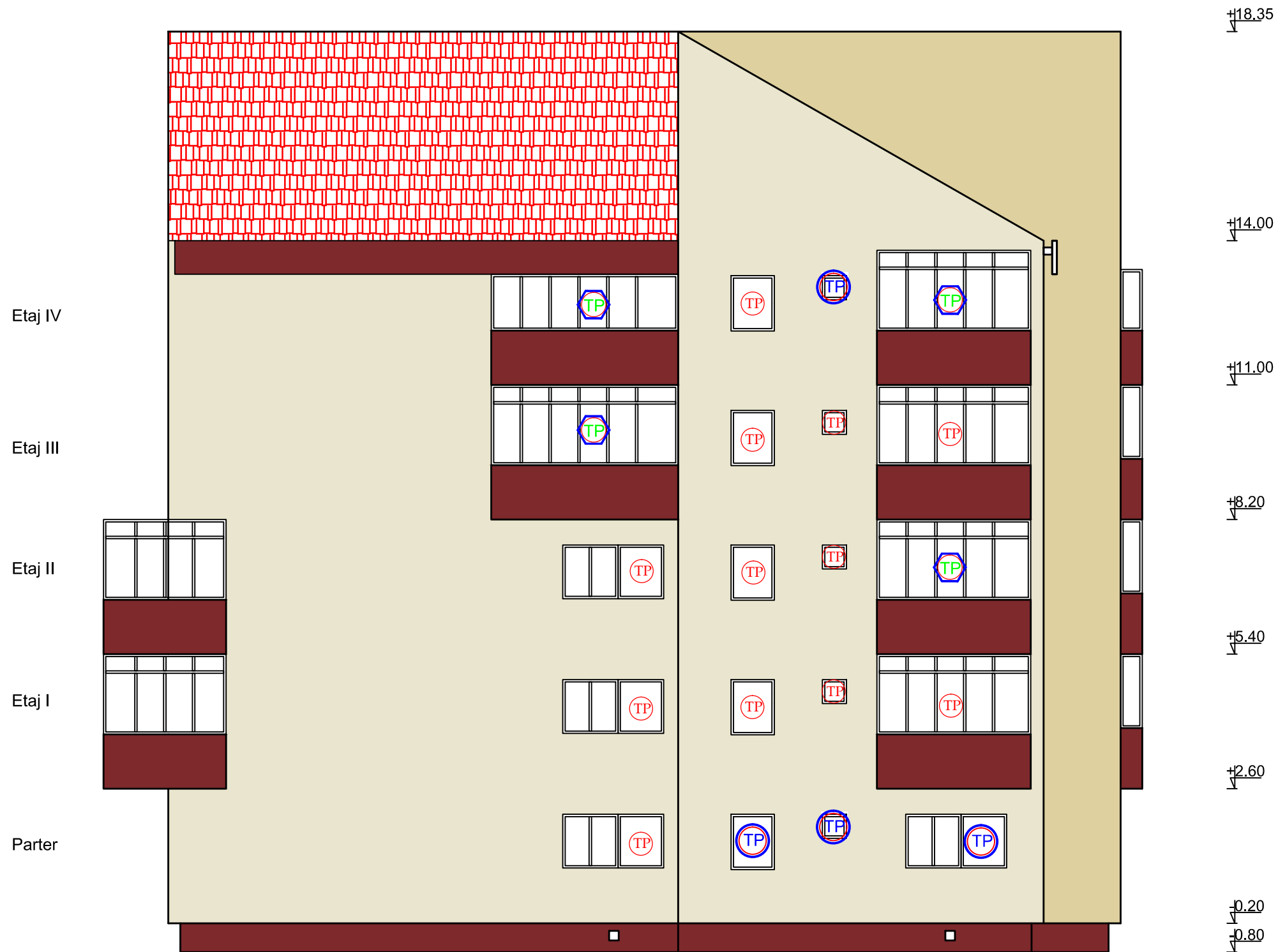
Fatada lateral dreapta propusa Scara 1:100
